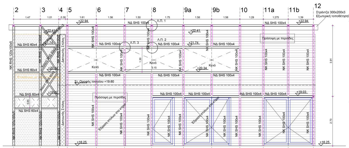
σχ.2 Νότια όψη μεταλλικού σκελετού
