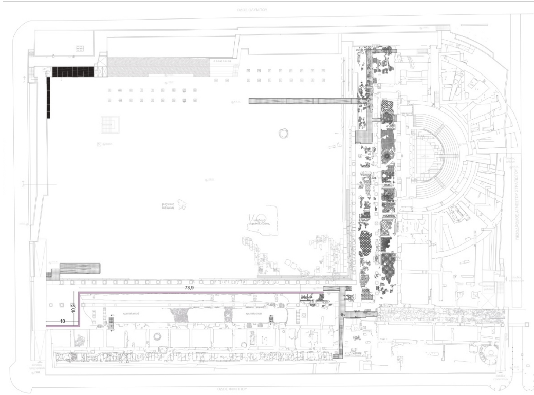
σχ.23 Κυκκλίδωμα νότιας στοάς – Κάτοψη
