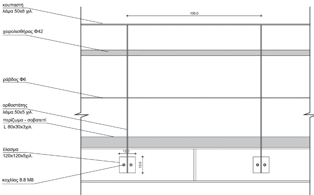
σχη.21 Κιγκλίδωμα μεταλλικών διαδρόμων - Όψη
