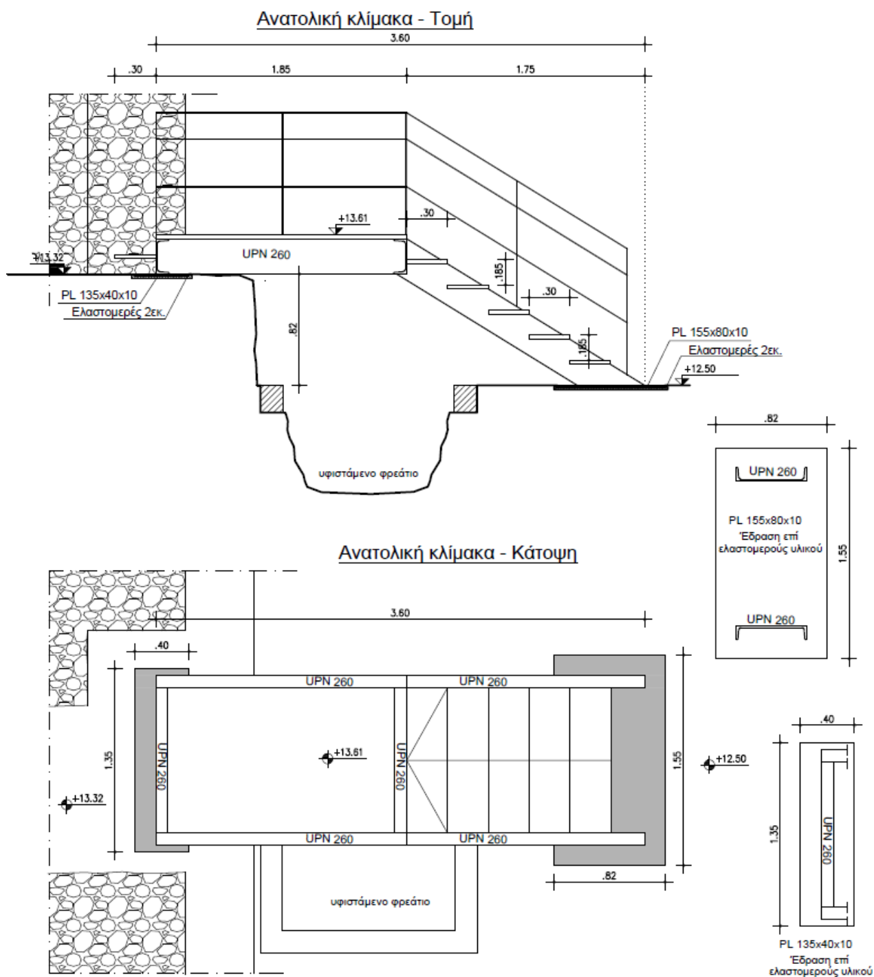
σχ.18β Ανατολική κλίμακα Κρυπτής Στοάς
