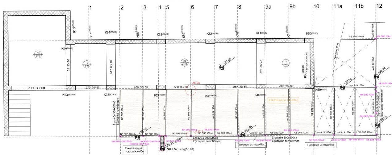
σχ.4 Κάτοψη στάθμης +22.94
