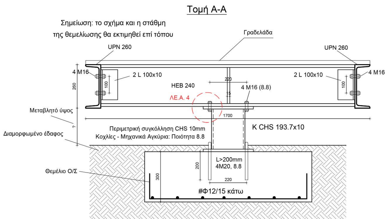
σχ.14 Εγκάρσια τομή (A-A) μεταλλικού διαδρόμου νοτιοανατολικά/βορειοανατολικά
