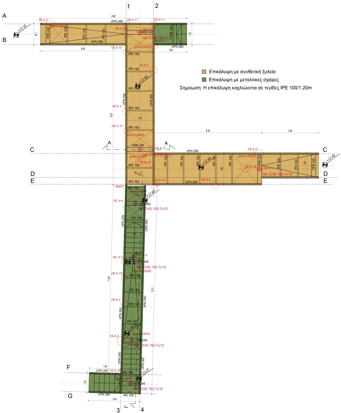
σχ.15 Κάτοψη μεταλλικού διαδρόμου νοτιοανατολικά
