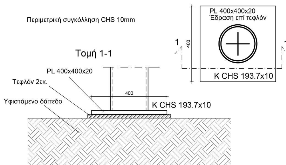
σχ.17 Έδραση στύλου επί ψηφιδωτού
