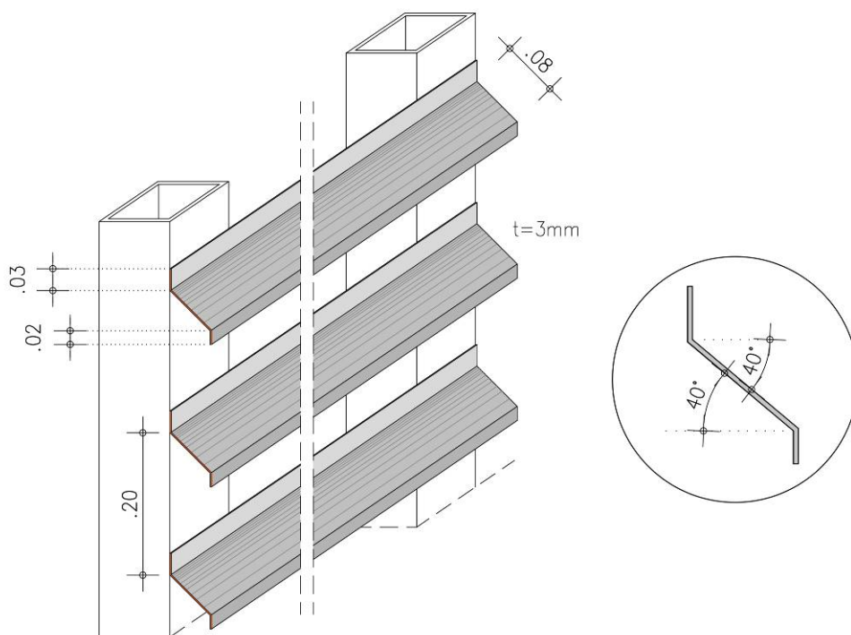
σχ.7 Περσίδες επικάλυψης όψεων
