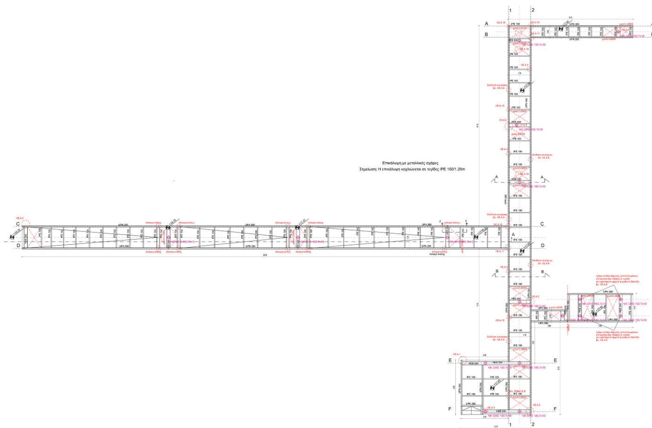
σχ.16 Κάτοψη μεταλλικού διαδρόμου βορειοανατολικά
