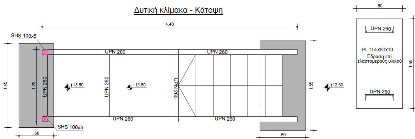
σχ.18α Δυτική κλίμακα Κρυπτής Στοάς
