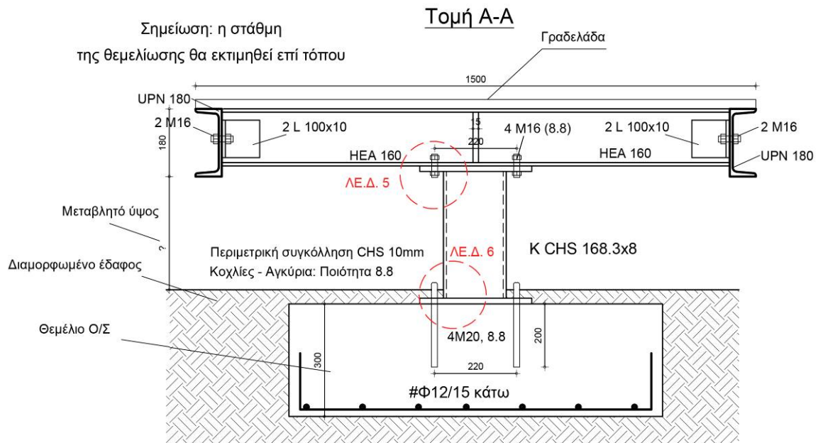
σχ.13 Εγκάρσια τομή (Α-Α) μεταλλικής ράμπας νοτιοδυτικά
