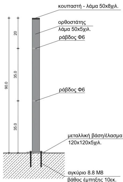
σχ.26 Κιγκλίδωμα νότιας στοάς – Τομή
