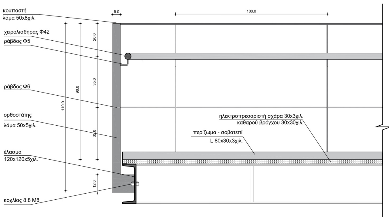
σχ.20 Κιγκλίδωμα μεταλλικών διαδρόμων - Τομή
