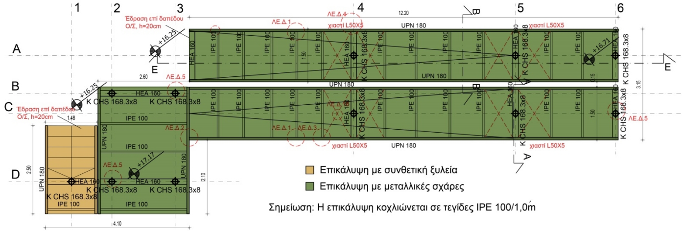
σχ.12 Κάτοψη μεταλλικής ράμπας νοτιοδυτικά
