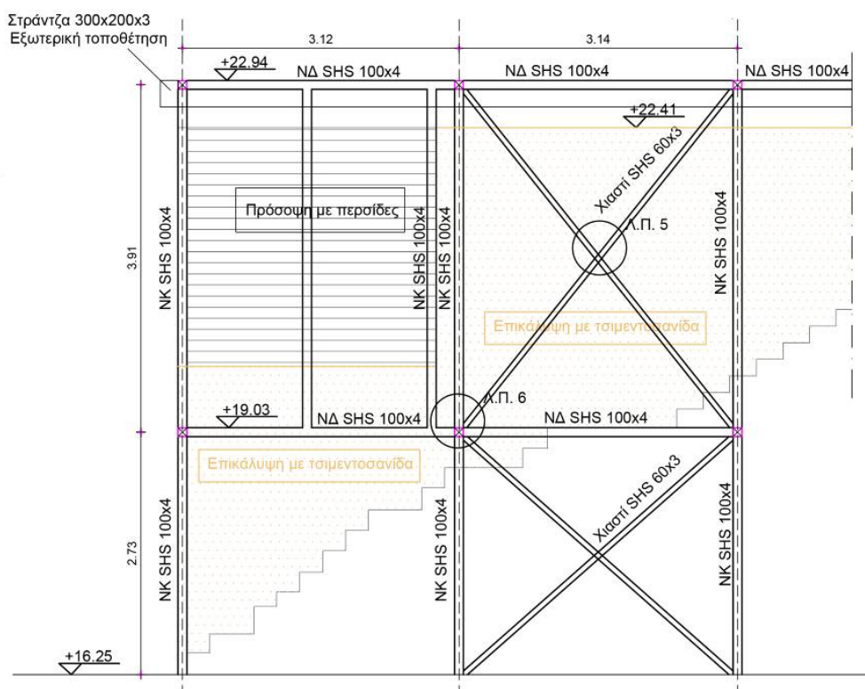
σχ.3 Ανατολική όψη μεταλλικού σκελετού
