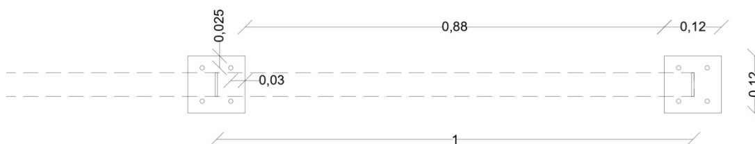
σχ.27 Κιγκλίδωμα νότιας στοάς – Οριζόντια τομή
