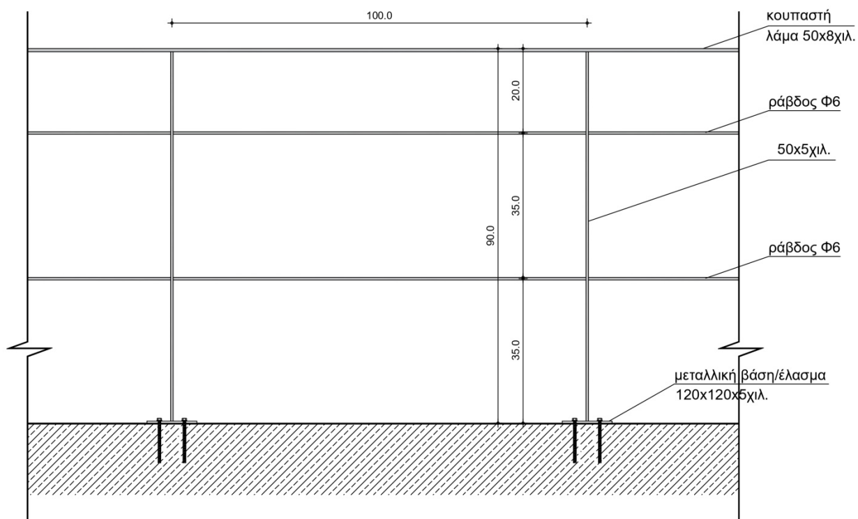
σχ.25 Κικκλίδωμα νότιας στοάς – Όψη
