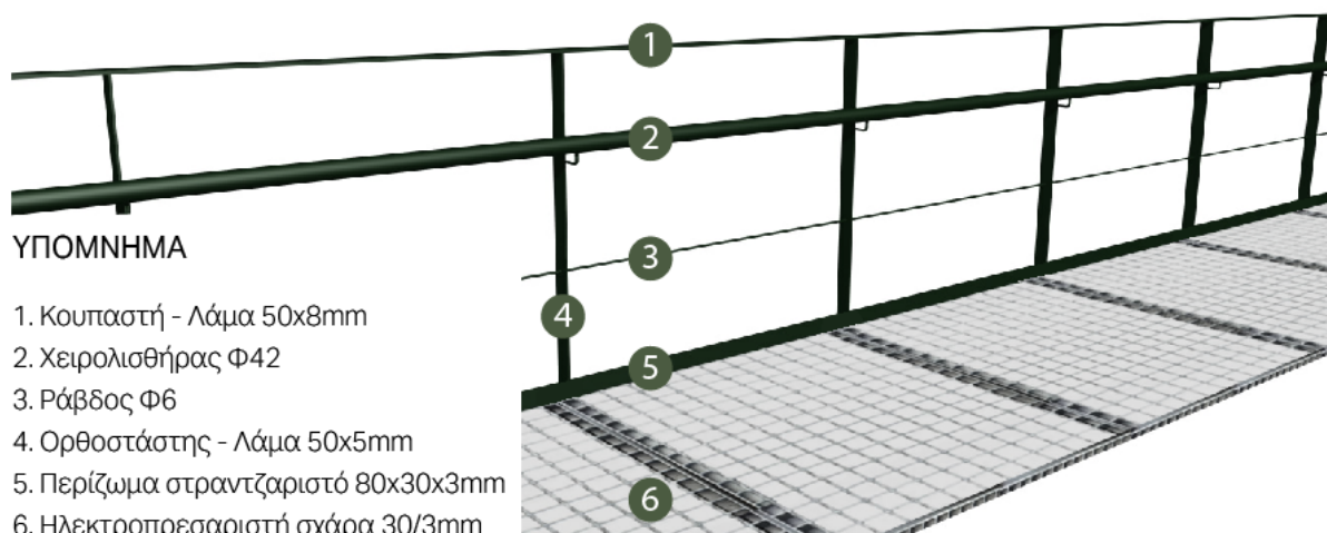
σχ.19 Κιγκλίδωμα μεταλλικών διαδρόμων
