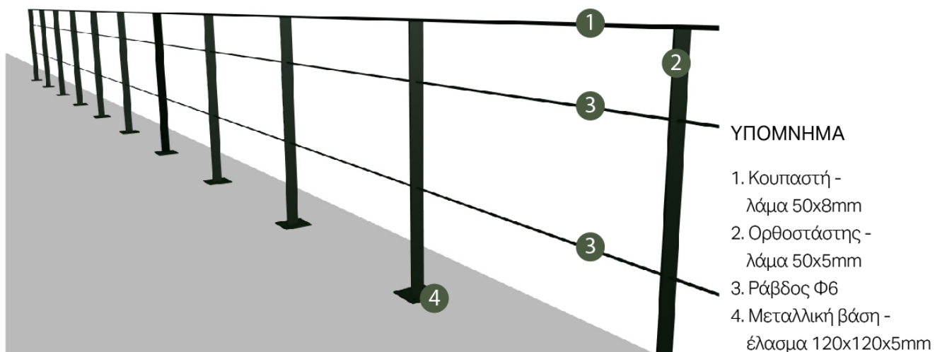
σχ.24 Κικκλίδωμα νότιας στοάς
