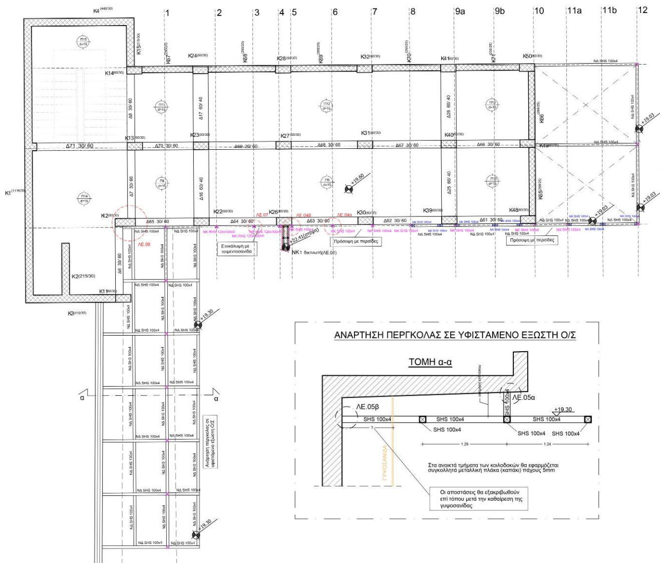
σχ.10 Κάτοψη στάθμης +19.30/+19.60
